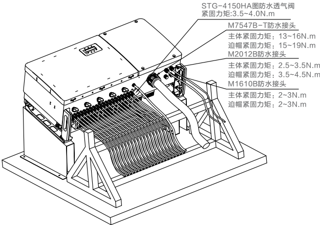
图3.24 扭矩参考
