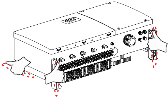
图3.4 逆变器手柄
