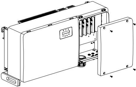
图3.21 拆下接线盒盖
