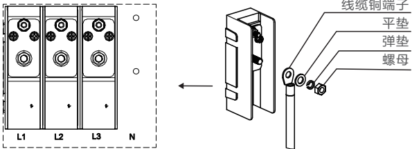
图3.20 铜铝过渡转接端子
