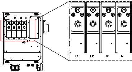
图3.22 带零线接线
