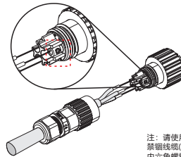
图 4.18 连接电缆线
