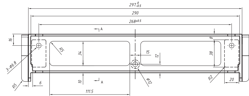
图4.3 背挂板尺寸
